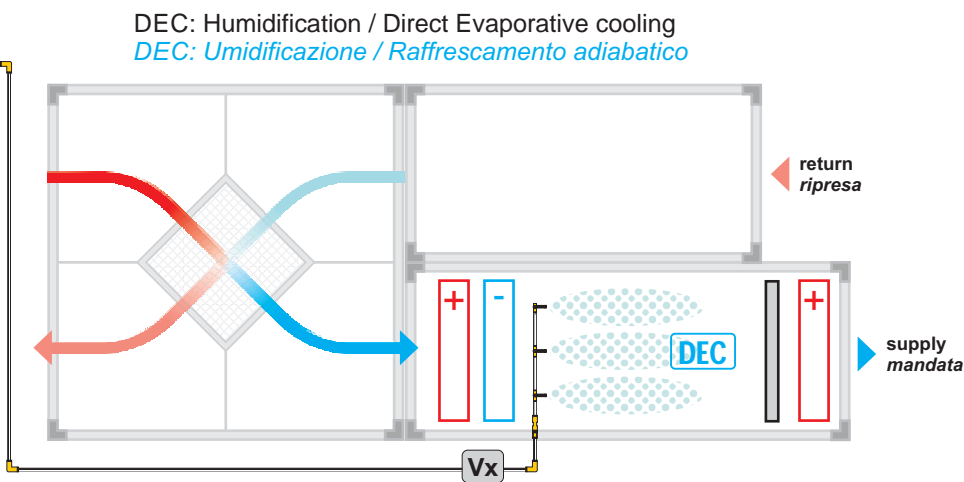
V = SOLENOID VALVES DRAIN KIT - ELETTROVALVOLE SCARICO
